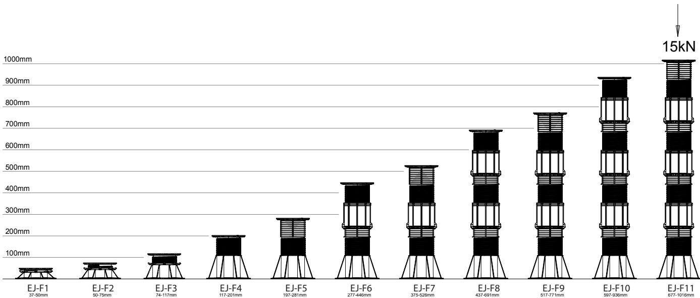
ECOJACK HEIGHT CHART
